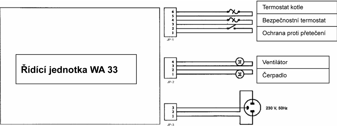
Obrázek 2 - Řídící jednotka - skupiny vodičů
