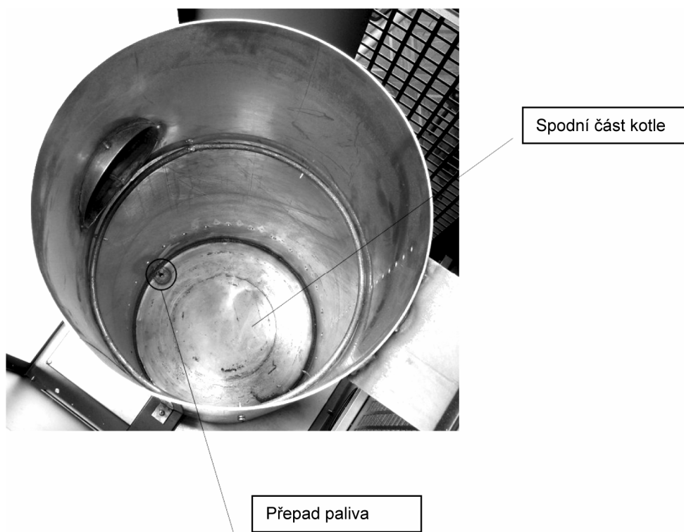
Obrázek 7 Spalovací komora
